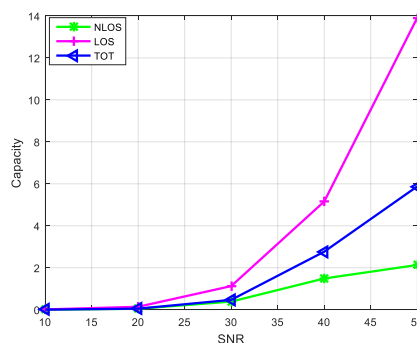
شکل ۳. مقایسه ظرفیت کانال ها بر حسب تغییرات SNR
