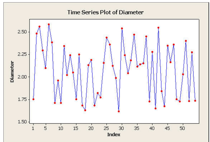
شکل 12- قطر ناگت بر اساس ترتیب انجام آزمایش ها
