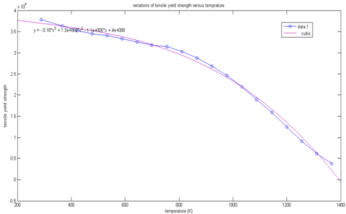
شکل 1- تغییرات تنش تسلیم Hastelloy X برحسب دما به صورت تابع درجه 3
