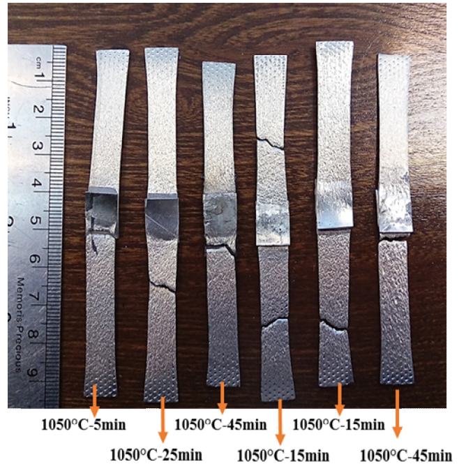
شکل 9. نمونه های اتصال داده شده اینکونل 600 بعد از آزمون استحکام برشی.
