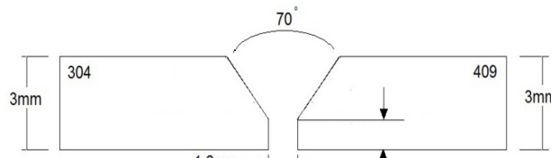
شکل 4- طرح اتصال نمونه های جوهرکاری شده
