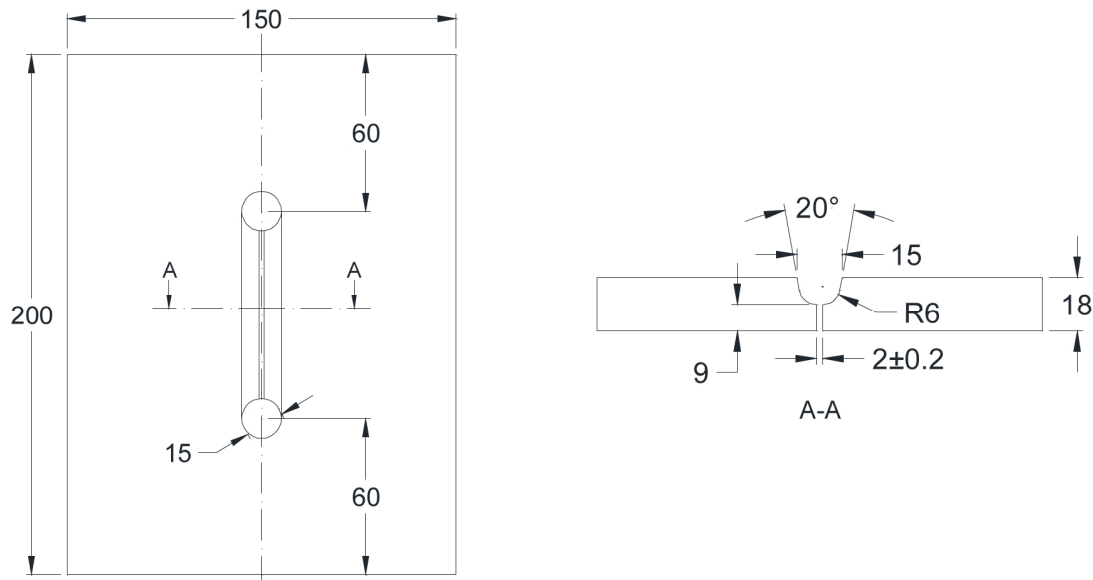
شکل 3- نمونه آماده شده از جنس فولاد X70 با شیار U برای آزمایش ترک سرد بر اساس استاندارد ISO17642-2 [19] (ابعاد بر حسب میلیمتر هستند)
