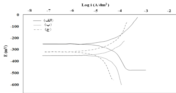
شکل 7- نمودارهای حاصل از آزمون خوردگی در مورد نمونه‌های جوشکاری شده در سه حرارت ورودی الف) 0/6، ب) 1/0 و ج) 1/4 کیلو ژول بر میلی متر.
