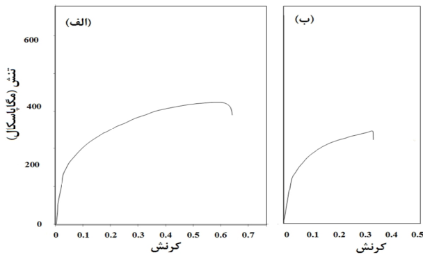
شکل 8- نمودارهای تنش - کرنش مهندسی نمونه‌های حاصل از جوشکاری و با انجام پیش‌گرمایش در دماهای الف) 50 و ب) 100 درجه سانتی‌گراد.
