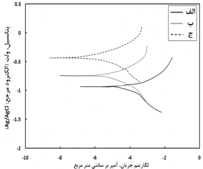
شکل 4- نمودارهای مربوط به آزمایش پلاریزاسیون پتانسیودینامیک با حداقل سه بار تکرارپذیری برای فلز جوش ایجاد شده با حرارت ورودی: (الف) 12/6 \text{ kJ/mm} ، (ب) 18/9 \text{ kJ/mm} ، (ج) 37/8 \text{ kJ/mm} .
