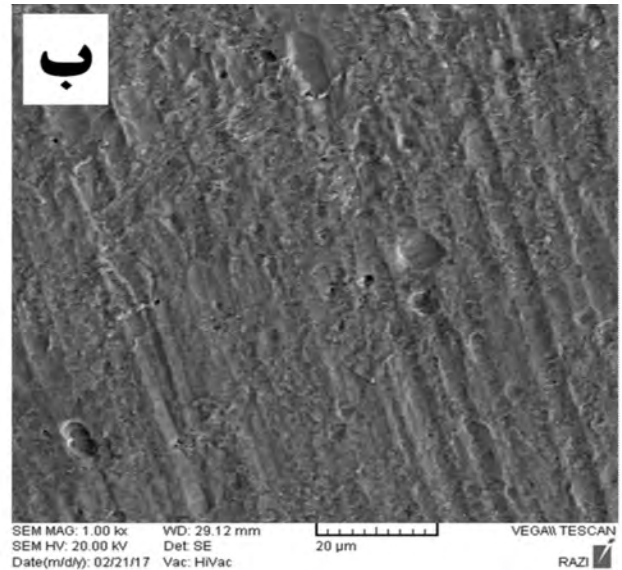
شکل 6- تصاویر میکروسکوپ الکترونی روبشی از سازوکار خوردگی فلز جوش ایجاد شده با حرارت ورودی: الف) ۱۲/۶ kJ/mm، ب) ۳۷/۸ kJ/mm
