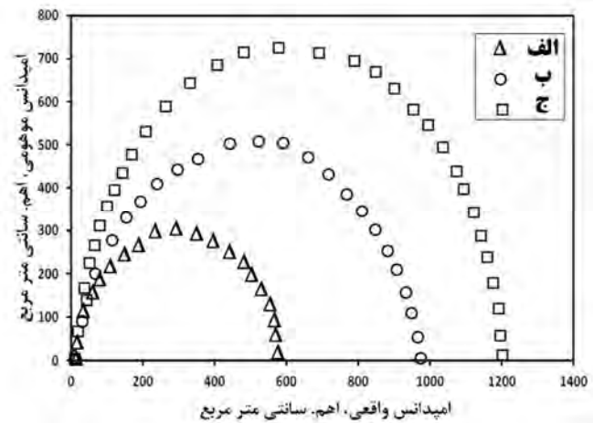
شکل 5- نمودار نایکویست مربوط به آزمایش طیف سنجی امپدانس الکتروشیمیایی با حداقل سه بار تکرارپذیری برای فلز جوش ایجاد شده با حرارت ورودی: الف) 12/6 kJ/mm، ب) 18/9 kJ/mm، ج) 37/8 kJ/mm
