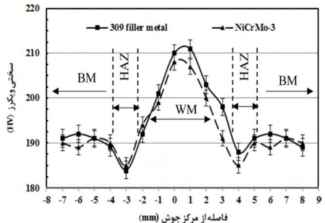
شکل 5- تاثیر ترکیب شیمیایی فلزپرکننده بر پروفیل سختی عمود بر مقطع جوش.
