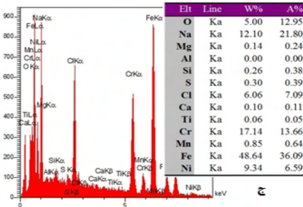
شکل 9- مطالعه سطح شکست خوردگی-خستگی نمونه جوشکاری شده با فلزپرکننده ER309L. (الف) تشکیل حفرات، (ب) تشکیل محصولات غنی از محیط خورنده، (ج) آنالیز EDS از ذرات M و N به ترتیب معرف حفرات و محصولات خوردگی در سطح شکست می‌باشد.
