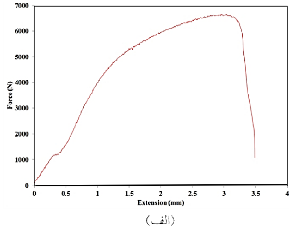
شکل (8). نمودار نیرو - جابجایی اتصالات مربوط به (الف) نمونه جوشکاری شده بدون لایه واسط و (ب) با حضور لایه واسط AISI347 (جریان جوشکاری برابر با 90 آمپر و مدت زمان عبور جریان 3 ثانیه).
