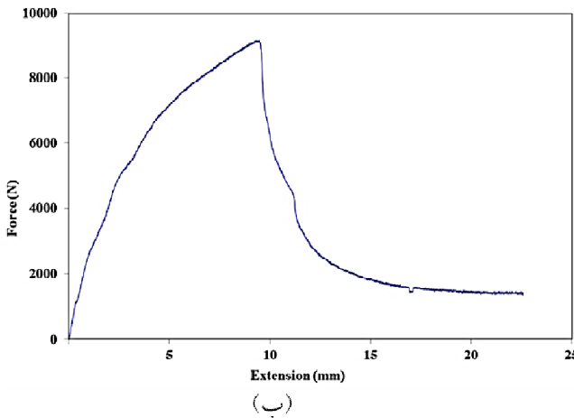
شکل (8). نمودار نیرو - جابجایی اتصالات مربوط به (الف) نمونه جوشکاری شده بدون لایه واسط و (ب) با حضور لایه واسط AISI347 (جریان جوشکاری برابر با 90 آمپر و مدت زمان عبور جریان 3 ثانیه).
