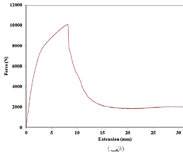
شکل 7- نمودار نیرو - جابجایی اتصالات با (الف) پیشینه (جریان جوشکاری برابر با 90 آمپر و مدت زمان عبور جریان 3 ثانیه) و (ب) کمینه (جریان جوشکاری برابر با 55 آمپر و مدت زمان عبور جریان 3 ثانیه) استحکام کششی - برشی مربوط به نمونه های جوشکاری شده بدون لایه واسط.
