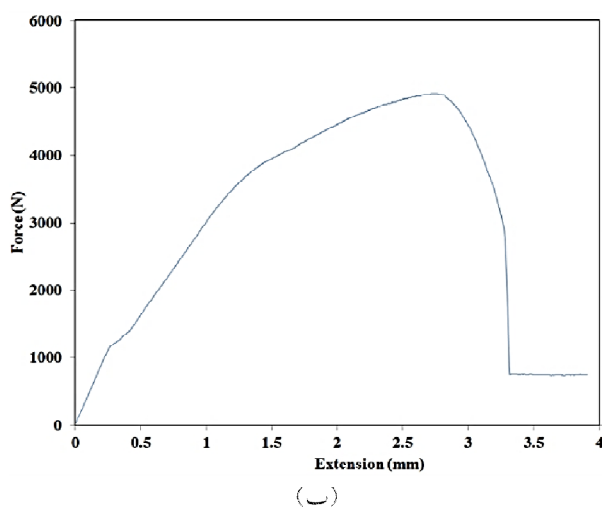
شکل 7- نمودار نیرو - جابجایی اتصالات با (الف) پیشینه (جریان جوشکاری برابر با 90 آمپر و مدت زمان عبور جریان 3 ثانیه) و (ب) کمینه (جریان جوشکاری برابر با 55 آمپر و مدت زمان عبور جریان 3 ثانیه) استحکام کششی - برشی مربوط به نمونه های جوشکاری شده بدون لایه واسط.
