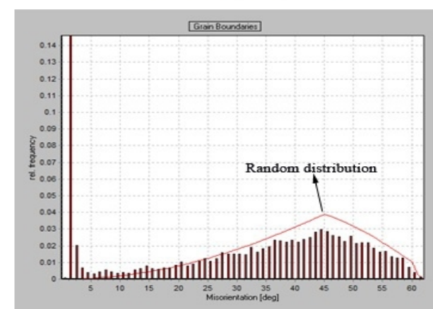
شکل 7- توزیع مرزانه های نانوکامپوزیت Al-4n6mAl_2O_3 جوشکاری شده با (الف) سرعت 1600rpm و سرعت خطی 32mm/min (ب) سرعت 1600rpm و سرعت خطی 40mm/min
