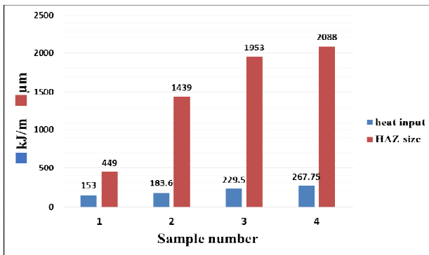
شکل ۸- مقایسه میانگین اندازه منطقه HAZ و گرمای ورودی عملی برای نمونه های جوشکاری
