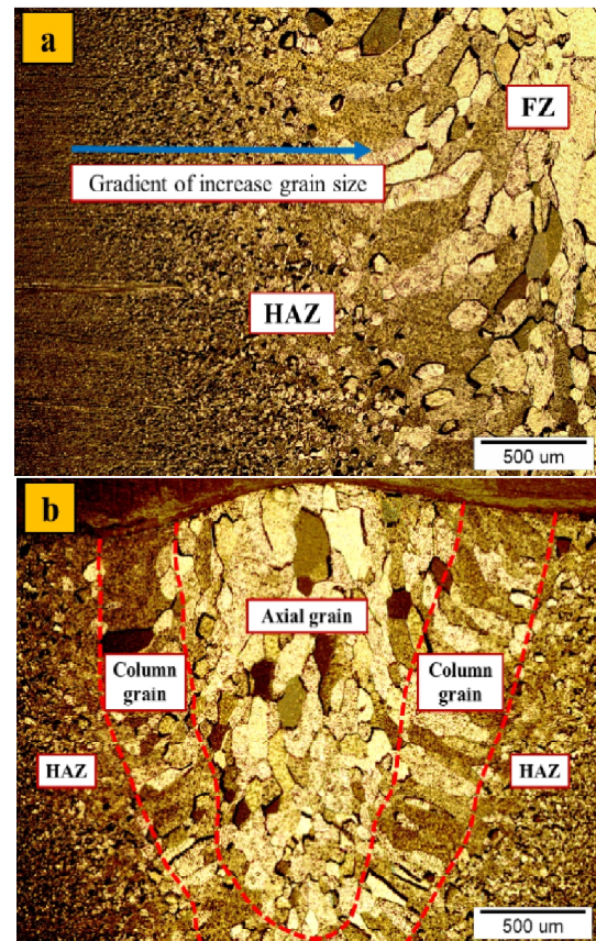
شکل ۵- ساختار میکروسکوپی مناطق جوشکاری پرتو الکترونی نمونه N2
