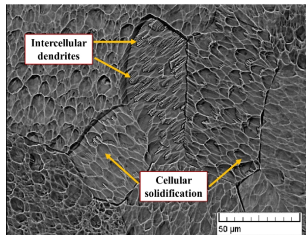
شکل ۷- تصویر میکروسکوپ الکترونی رویشی از مرکز جوش
