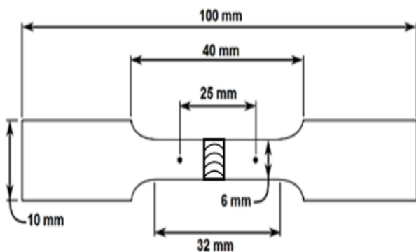
شکل 1- ابعاد نمونه کشش بر اساس استاندارد ASTM.E8/E8M
