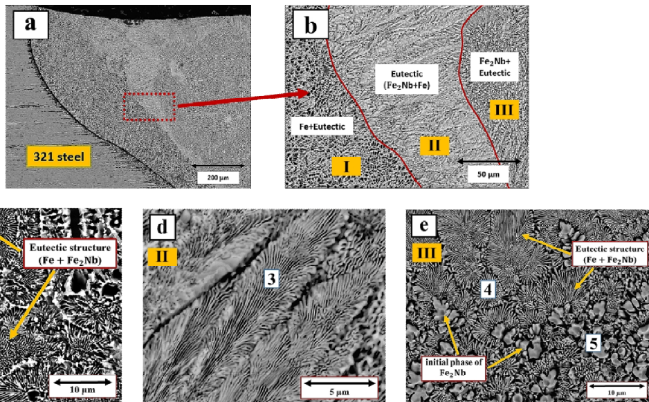
شکل ۱۰- تصویر ریزساختار میکروسکوپ الکترونی روبشی از اتصال غیر هم جنس Nb-1Zr به فولاد
