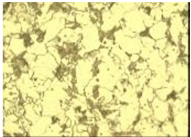
شکل 11- تصاویر میکروسکوپی ناحیه متأثر از حرارت مجاور جوش
