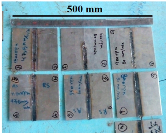
شکل 5- چند نمونه از اتصالات سالم و معیوب مطابق پارامترهای شکل (4)
