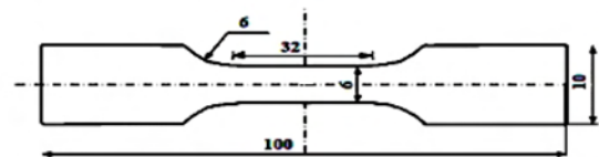
شکل 3- نمونه آزمایش کشش، طبق استاندارد ASTM E8.
