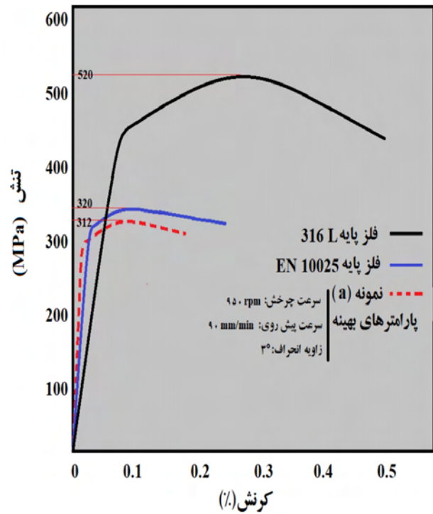
شکل 22- نمودار تنش کرنش. فلزات پایه و نمونه جوش خورده با پارامترهای بهینه.
