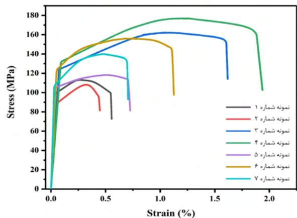
شکل ۶- منحنی‌های تنش-کرنش نمونه‌های جوشکاری شده.
