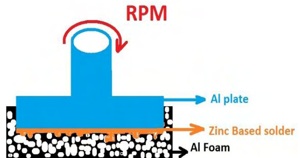
شکل 1- شماتیک ابزار چرخشی با قطر 35 \text{ mm} قابل چرخش همراه لحیم پایه روی در حوضچه تعبیه شده در فوم آلومینیوم.
