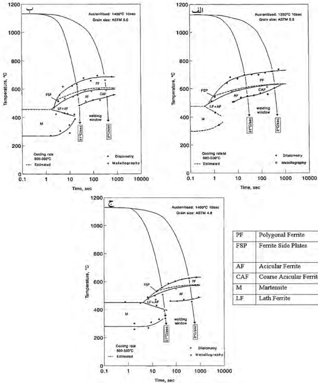
شکل 1- تاثیر افزایش نیکل بر نمودارهای CCT مربوط به فلزجوش های C-Mn-Ni (الف) C=0.05%, Mn=1.2%, Ni=1.1%
