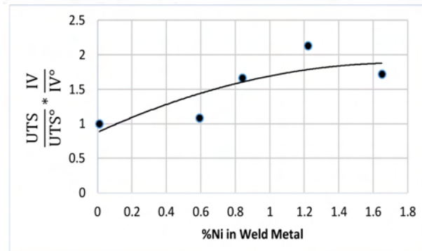
شکل ۱۰- تغییرات پارامتر حاصلضرب استحکام کششی نرماله شده (\frac{UTS}{UTS^0}) در انرژی ضربه نرماله شده (\frac{IV}{IV^0}) بر حسب مقدار نیکل موجود در فلزجوش.
