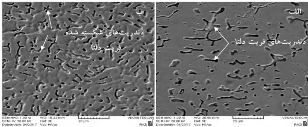
شکل ۶- تصاویر SEM از فلز جوش ER309L الف- بدون لرزش و ب- با لرزش تحت ولتاژ ۳۰ ولت
