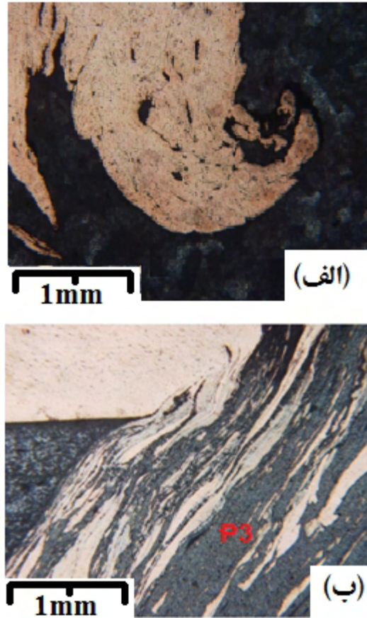
شکل ۹- ساختار لایه ای شکل گرفته با ابزار (الف) رزوه ای و (ب) ساده
