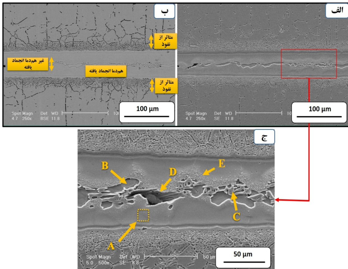
شکل ۶- تصاویر میکروسکوپی الکترونی روبشی از ریزساختار ناحیه اتصال فاز مایع گذرا در دمای ۱۰۵۰ درجه سانتیگراد و زمان ۵ دقیقه (الف) الکترونهای ثانویه، (ب) الکترون های برگشتی، (ج) تصویر با بزرگنمایی بالا از منطقه انجماد همدمما و غیرهمدمما نشان دهنده حضور فازهای مختلف،
