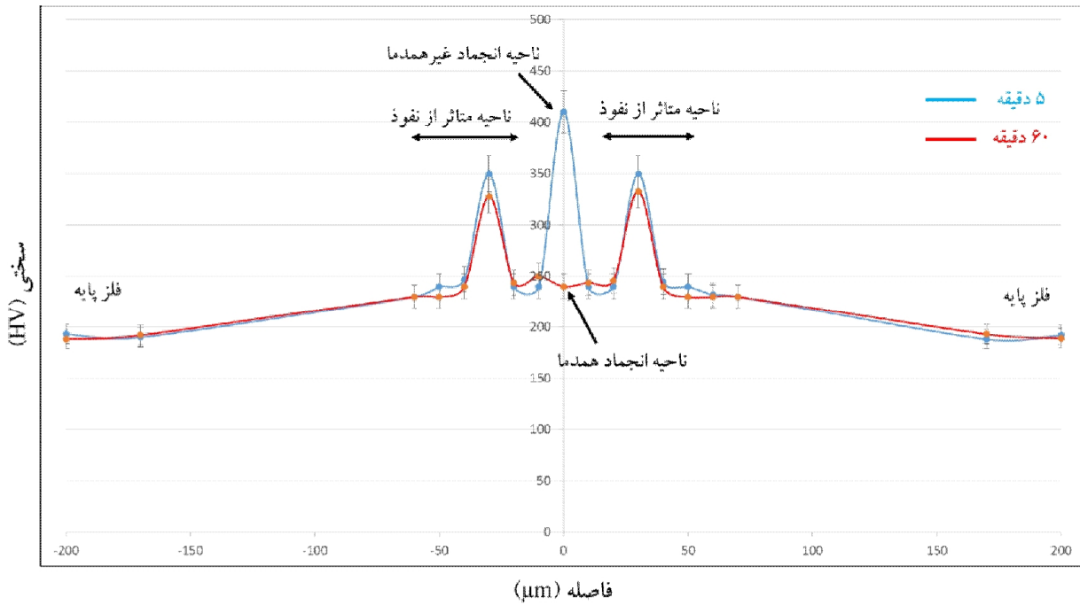
شکل ۱۰- پروفیل ریزسختی سنجی اتصالات بدست آمده در دمای 1050^{\circ}\text{C} و زمان‌ها ۵ و ۶۰ دقیقه
