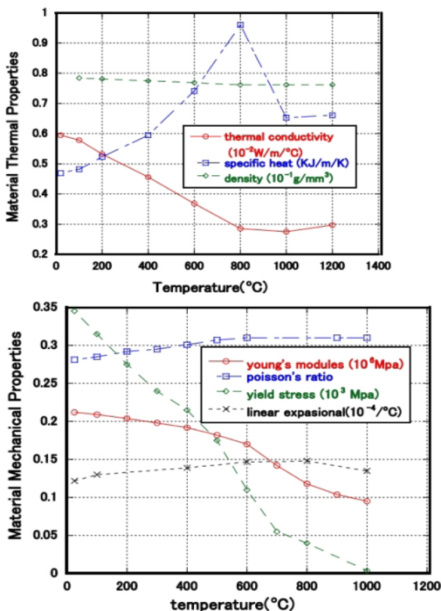
شکل 3- خواص مواد وابسته به دما برای فولاد اس ام 490 [13]
