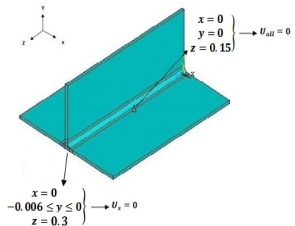
شکل 6- شرایط مرزی مکانیکی
