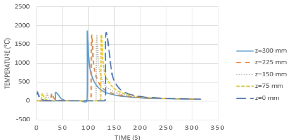
شکل 8- نمودار دما - زمان در نقاط مختلف محل جوشکاری
