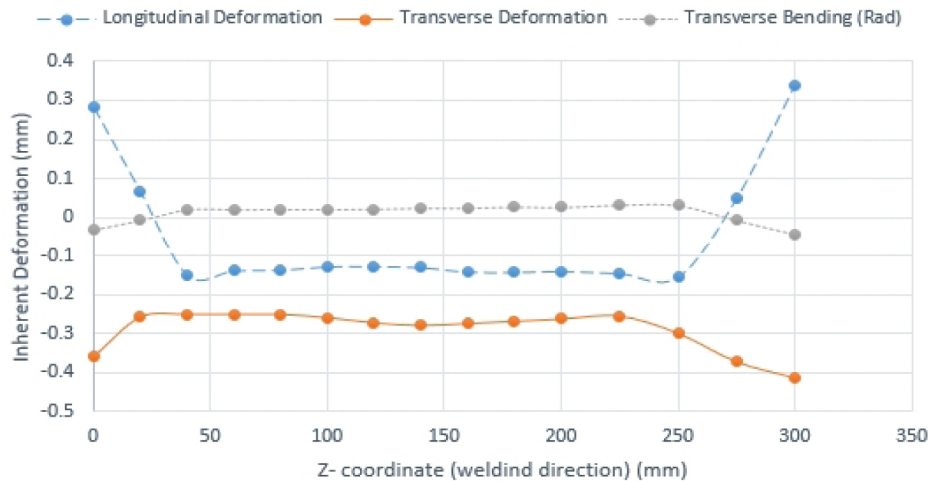
شکل 7- توزیع تغییر شکل های ذاتی در جهت خط جوش
