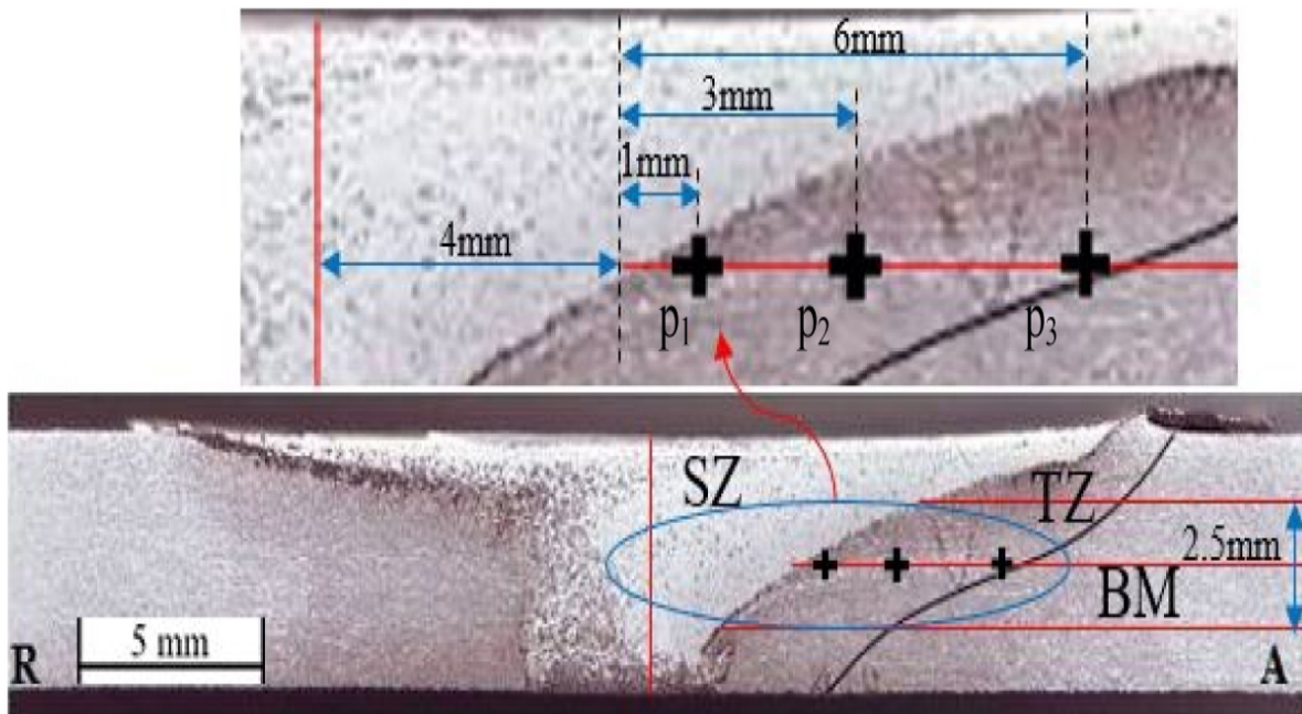
شکل 2- فواصل سوراخ های تعبیه شده نسبت به ناحیه اغتشاش در مقطع ماکروساختار.
