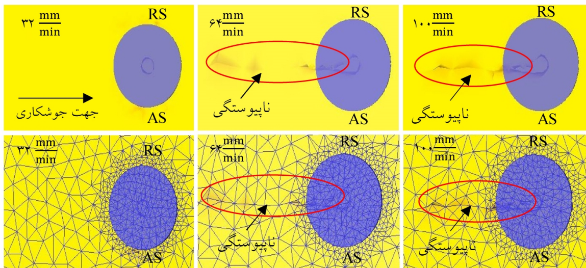
شکل 13- مقایسه کیفیت اتصالات جوشی در سرعت های پیشروی مختلف (32، 64 و 100 mm/min).
