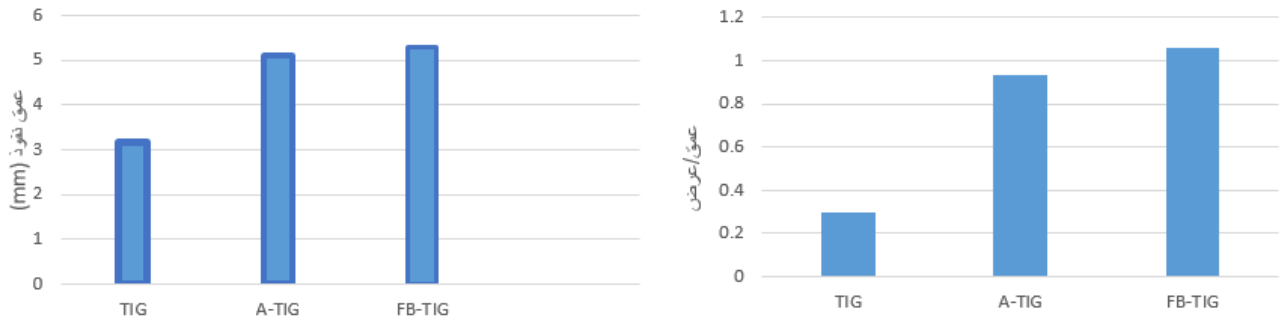
شکل ۷- مقایسه عمق نفوذ و نسبت عمق به عرض جوش در روش‌های TIG، A-TIG و FB-TIG
