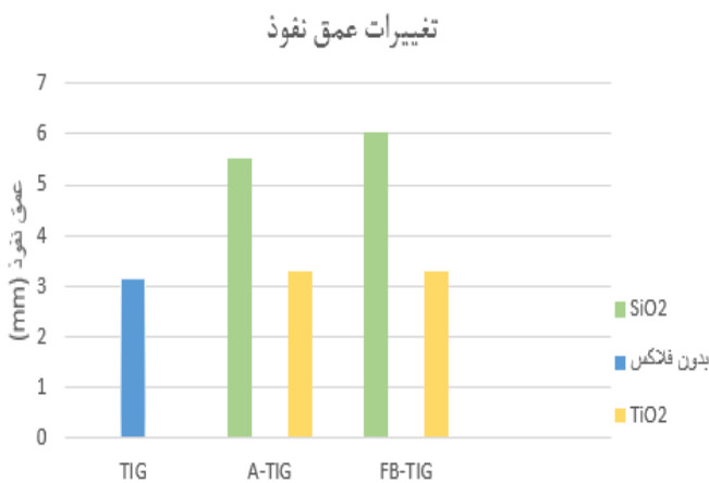
شکل 4- نمودارهای مقایسه عمق نفوذ و نسبت عمق به عرض نمونه‌های مرحله اول
