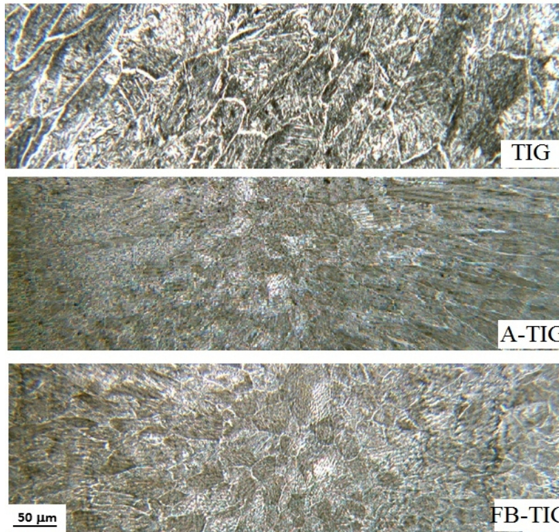
شکل ۸- تصاویر میکروسکوپی تهیه شده از ریزساختار جوش نمونه‌های جوشکاری شده به سه روش TIG، A-TIG و FB-TIG
