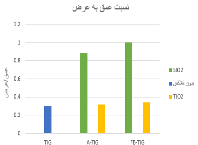
شکل 4- نمودارهای مقایسه عمق نفوذ و نسبت عمق به عرض نمونه‌های مرحله اول
