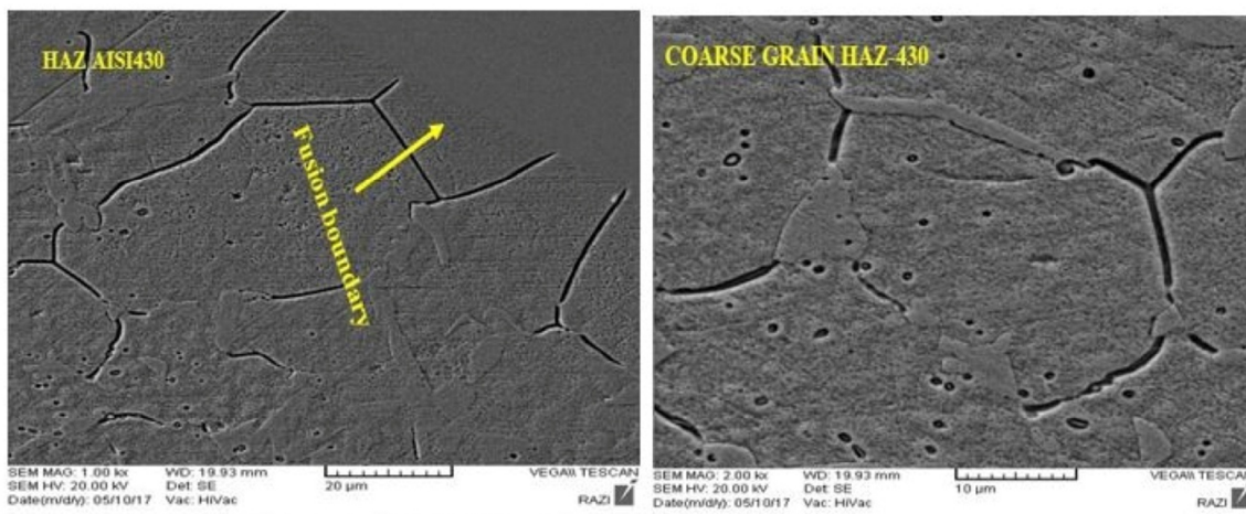
شکل 8- تصویر میکروسکوپی نوری از ریزساختار HAZ فلز پایه فولاد زنگ نفریتی 430 با فلز جوش (نمونه حرارت ورودی کم).
