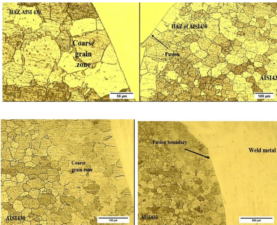
شکل 7- تصویر میکروسکوپی نوری از ریزساختار منطقه HAZ فلز پایه فولاد زنگ نفریتی با فلز جوش.
