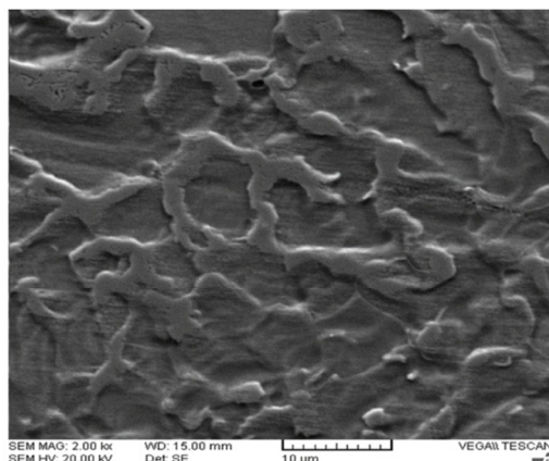
شکل 15- تصویر میکروسکوپی الکترونی روبشی از منطقه HAZ فلز پایه اینکونل 625 و فلز جوش .
