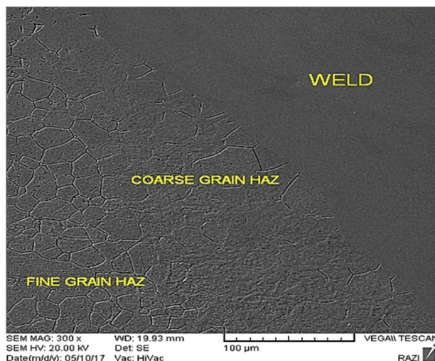
شکل 9- تصویر میکروسکوپی الکترونی روبشی و طیف نگاری آنالیز عنصری EDS از منطقه HAZ ریزساختار فولاد زنگ‌نزن فریتی 430 با فلز جوش.
