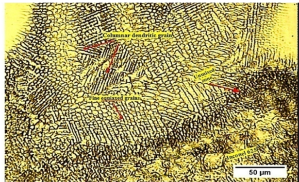
شکل 12- تصویر میکروسکوپ نوری از ریز ساختار فصل مشترک فلز پایه اینکونل 625 با فلز جوش.
