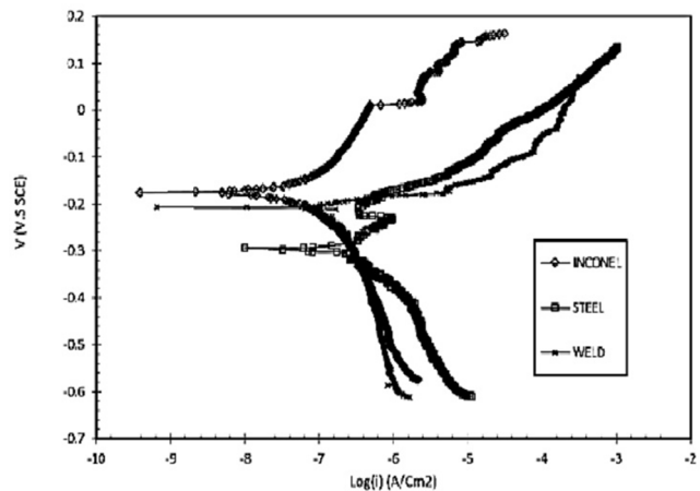
شکل 20- مقایسه نمودار پلاریزاسیون تافل نمونه های اتصال و فلزات پایه.
