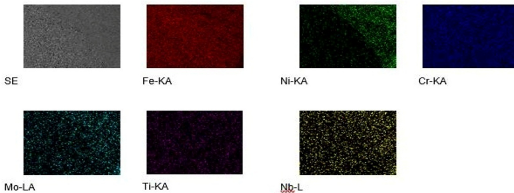
شکل 19- تصویر زمینه HAZ، فصل مشترک، فلز جوش، فلز پایه اینکونل 625 با نقشه عناصر Fe و Ni, Cr, Mo, Ti.
