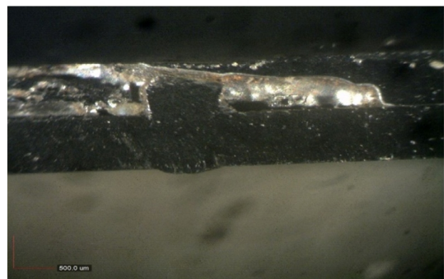
شکل 21- تصویر میکروسکوپی نوری از نمونه بهینه جوشکاری شده بعد از تست خوردگی.
