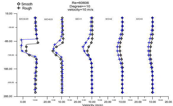
شکل ۱۱- تغییرات دنباله سرعت در دو حالت صاف و زبر در زاویه 10^\circ در Re = 60606
