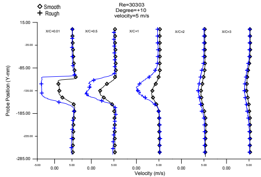
شکل ۷- تغییرات دنباله سرعت در دو حالت صاف و زبر در زاویه 10^\circ در Re=20303
