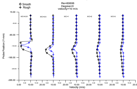
شکل ۹- تغییرات دنباله سرعت در دو حالت صاف و زبر در زاویه صفر درجه در Re=60606
