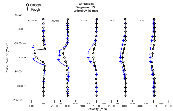
شکل ۱۲- تغییرات دنباله سرعت در دو حالت صاف و زبر در زاویه 15^\circ در Re = 60606
