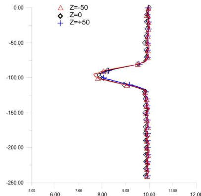
شکل ۴- دنباله جریان در سرعت ۱۰ متر بر ثانیه در X/C=2 در سه نقطه +50 و صفر و -50
