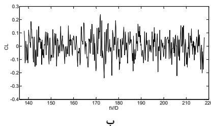
شکل ۸- الف نمودار نوسانات CL استوانه برای S = 0.1 و ب برای S = 0.2 که هر دو در L/D = 2.5, G = 2.5D و E_b^* = 0.001 و Re = 100 هستند
