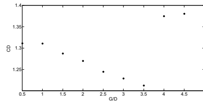
شکل ۱۰- نمودار تغییرات ضریب پسای استوانه با فاصله گرفتن لبه‌ی حمله رشته از استوانه در L/D = 4 و S = 0.1 و E_b^* = 0.0001 و Re = 100
