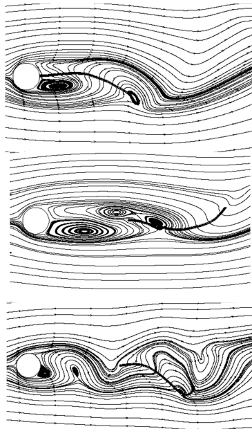
شکل ۱۱- نمای گردابه پشت استوانه در حضور رشته در S = 0.1 ، Re = 100 و E_b^* = 0.0001 و L/D = 4
