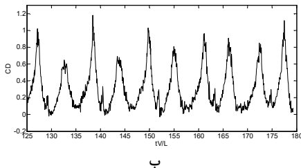
شکل ۹- نمودار پستی رشته در S = 0.1 و الف- در جریان آزاد، ب- در وضعیت پشت استوانه، که هر دو در L/D = 2.5, G = 2.5D و Re = 100 و E_b^* = 0.0001 هستند
