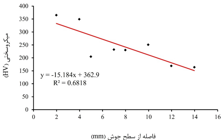
شکل ۱۳- پروفیل سختی
