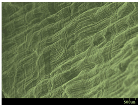
شکل ۹- نمایی از تقسیم بندی در سطح تراشه در سرعت ۶۰ متر بر دقیقه و نرخ پیشروی ۰.۲۵ میلیمتر بر دقیقه در حالت روانکاری کمینه
