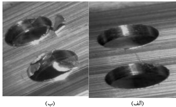
شکل ۱۴- شکل پلیسه‌های تولیدی در حالات (الف)سوراخکاری خشک و (ب)روانکاری کمینه
