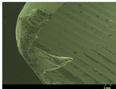
شکل ۱۰- سایش ابزار در حالت سوراخکاری خشک
