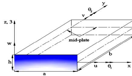
شکل ۲- ورق مستطیلی و دستگاه مختصات آن
