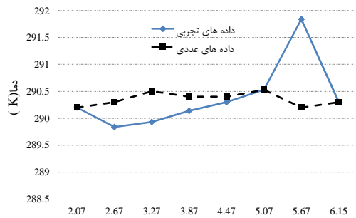
شکل ۹- نتایج مطالعه عددی و نتایج تجربی
