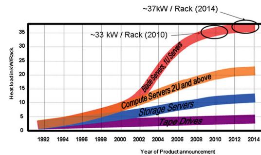
شکل ۱- روند تولید گرما در تجهیزات ارتباطاتی [۱]
