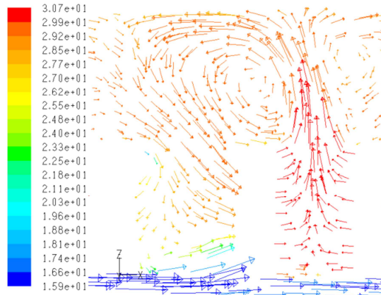
شکل ۱۶- بردارهای سرعت بر اساس دمای کل در محدوده راهروی گرم نشان دهنده پدیده چرخش هوای گرم اطراف راک
