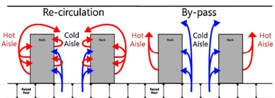
شکل ۳- چرخش هوای گرم و برگشت هوای سرد [۱۰]
