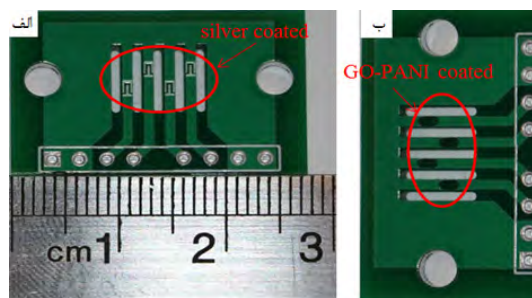
شکل ۳: الکترودها با پوشش نقره (الف) و الکترودها آماده شده (ب)
