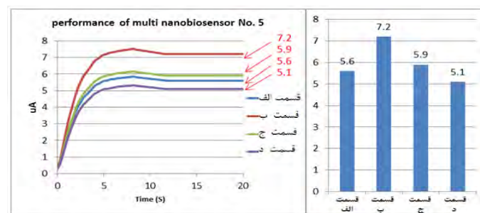
شکل ۱۱: نمودار پاسخ هر ۴ جزء نانوحسگر زیستی چندگانه به مخلوطی از ۲۰ ppm گاز اتانول، ۱۰ ppm گاز متان، ۵ ppm گاز آمونیاک و بدون گاز دی اکسید کربن
