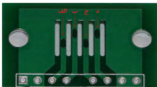
شکل ۲: هر الکترودها آماده شده دارای ۴ مکان مشخص شده با حروف الف، ب، ج و د است
