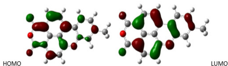
شکل ۱۰: تصاویر سطوح اوربیتال های مولکولی ماده رنگزای سنتز شده
