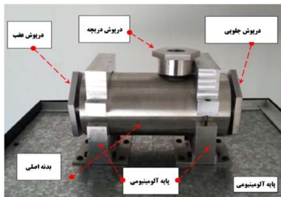
شکل ۶- استرنده برنر [۱۷].
