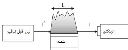
شکل (۲): نمودار شماتیک طیف جذبی [۹].
