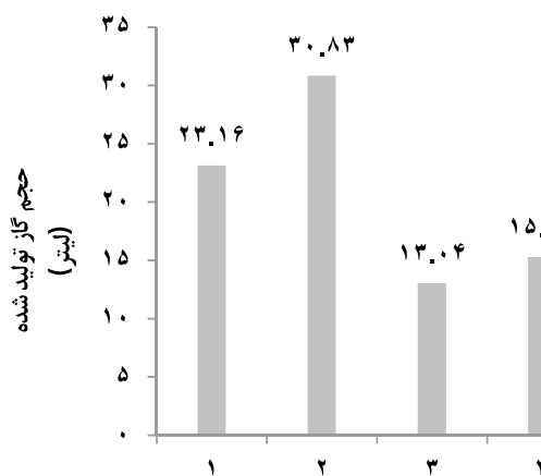
شکل ۴ نمودار ترکیب-حجم کود گاو‌میش و کلش ذرت
