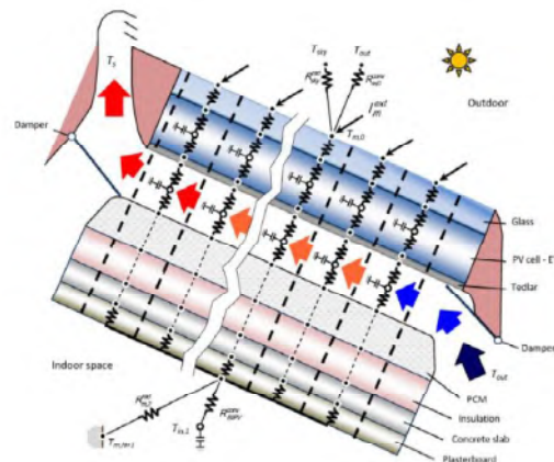
شکل ۲. پنل فتوولتائیک حرارتی به کار رفته در ساختمان مدل شده توسط Buonomano [16]
