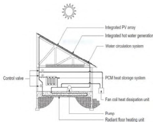
شکل ۳. سیستم ترکیبی خورشیدی با استفاده از مواد تغییر فاز دهنده و پنل فتوولتائیک برای ساختمان [۱۹]
