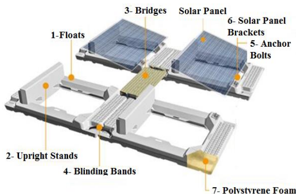
شکل ۳ یک سازه فوتوولتائیک شناور [۳]
