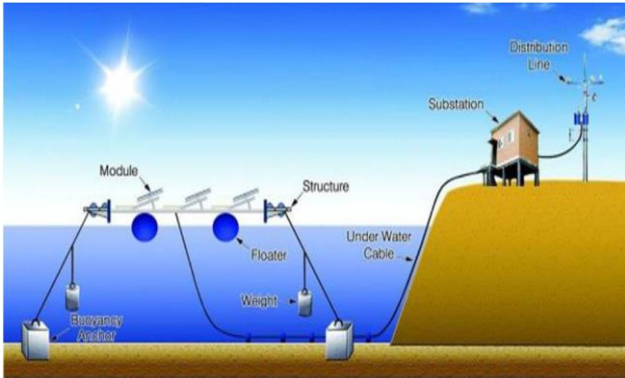
شکل ۲ طرح سیستم فوتوولتائیک خورشیدی شناور [۲]
