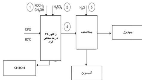
شکل ۸. نمایش شماتیک از فرایندهای تبدیل روغن پالم به بیودیزل [۴۱]
