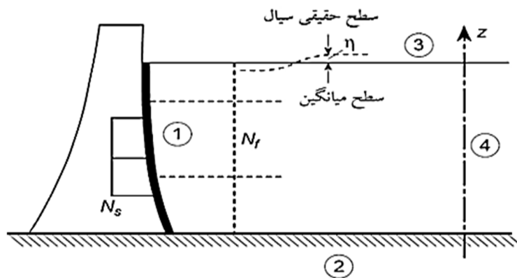
شکل ۴. انواع شرایط مرزی سیال [۲۹]
