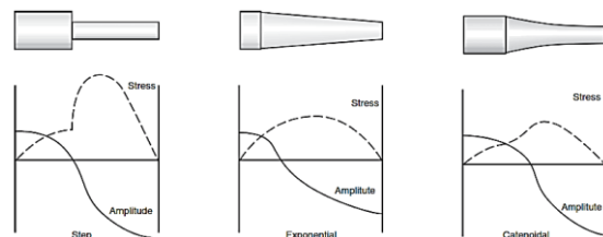
شکل ۷. پروفیل‌های مختلف هورن جوشکاری فراصوتی به همراه
