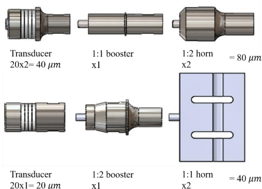
شکل ۴. افزایش دامنه ارتعاشات مبدل توسط بوستر و هورن
