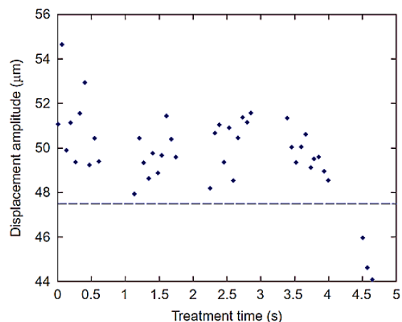
شکل ۸. نمایش دامنه حاصل از اعمال فراصوت در طول زمان با
