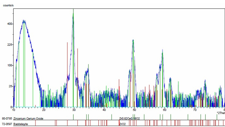
شکل ۳- نمونه ۲: زیرکونیای پایدار شده با سریم در دمای ۱۵۵۰ درجه سانتیگراد [۴].
