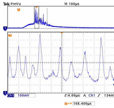
شکل ۸- پهنای پالس‌های زمانی لیزری کمتر از ۳ میکروثانیه
