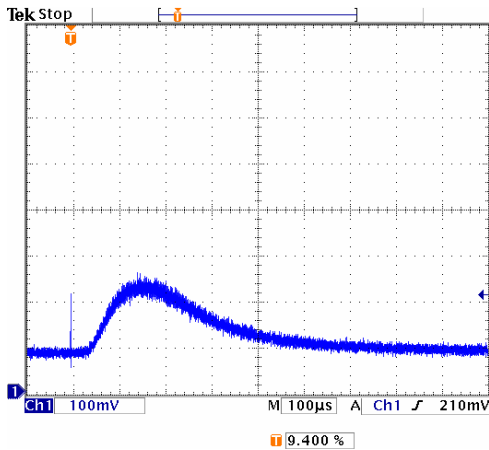
شکل ۹- پهنای پالس زمانی لامپ پس از مسدود کردن آینه عقب
