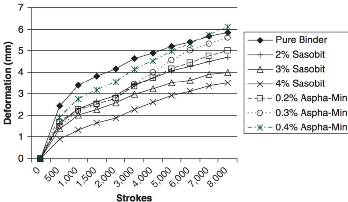
شکل ۲. نتایج عمق شیار برای PG ۶۴-۲۲
