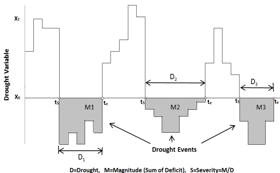
شکل ۲. ویژگی‌های خشکسالی با استفاده از تئوری دنباله‌ها (Yevjevich, 1967)
