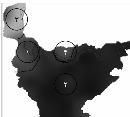
شکل ۳- پهنه‌بندی فرسایش‌پذیری با ۵ خوشه، خوشه‌های ۳، ۴ و ۵ به هم پیوسته شده‌اند
