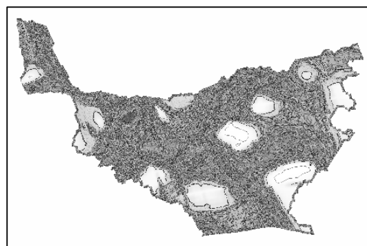
شکل ۶- نمایش سه‌بعدی کلاسهای ۳، ۴ و ۵ در حوضه (کلاسها به هم پیوسته شده‌اند)
