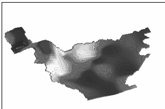
شکل ۴- نمایش سه‌بعدی کلاس ۱ در حوضه
