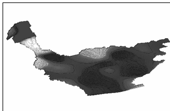
شکل ۵- نمایش سه‌بعدی کلاس ۲ در حوضه
