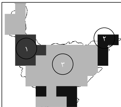
شکل ۱- پهنه‌بندی فرسایش‌پذیری، روش PSIAC
