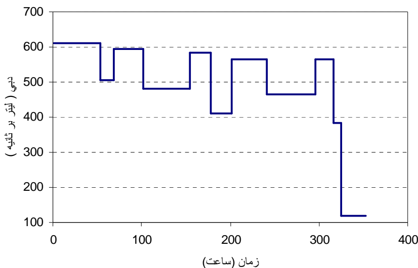
شکل ۶- هیدروگراف تنظیمات درجه سراب کانال برای گزینه یک
