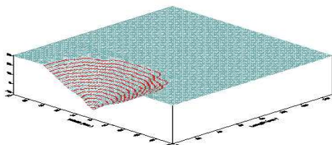
شکل ۴ ب - نمای سه‌بعدی از مخروط رسوب‌شویی پس از انجام آزمایش با دبی ۳ لیتر در ثانیه و ارتفاع آب ۹۰ سانتی‌متر
