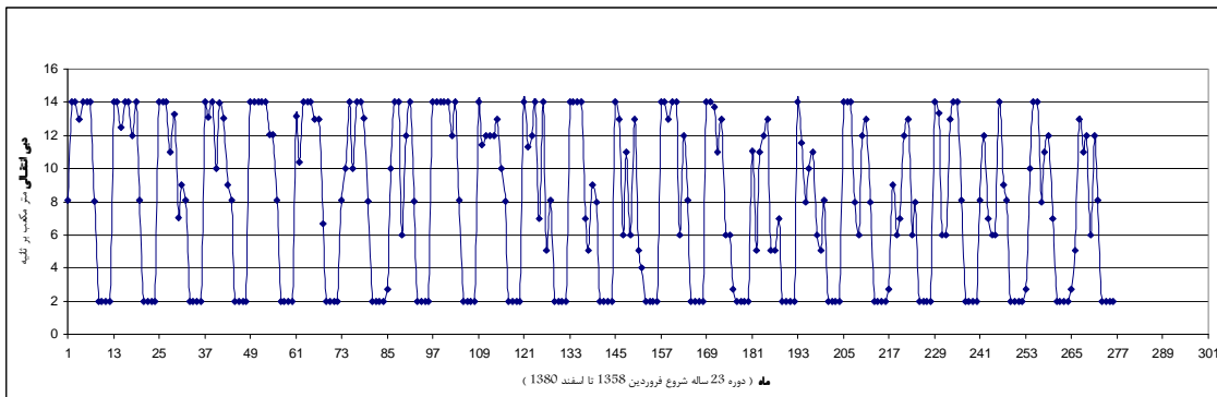
شکل ۱۰- دبی بهینه ماهانه انتقال در طول دوره بهینه‌سازی از تونل سولگان
