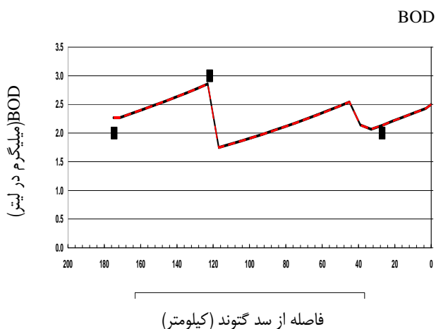
شکل ۷- مقادیر مشاهداتی و شبیه‌سازی دبی، EC، BOD و DO با استفاده از مدل شبیه‌سازی Qual2k در ماه فروردین در فاصله ایستگاه‌های گتوند- زرگان در رودخانه کارون
