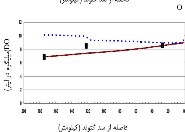
شکل ۷- مقادیر مشاهداتی و شبیه‌سازی دبی، EC، BOD و DO با استفاده از مدل شبیه‌سازی Qual2k در ماه فروردین در فاصله ایستگاه‌های گتوند- زرگان در رودخانه کارون
