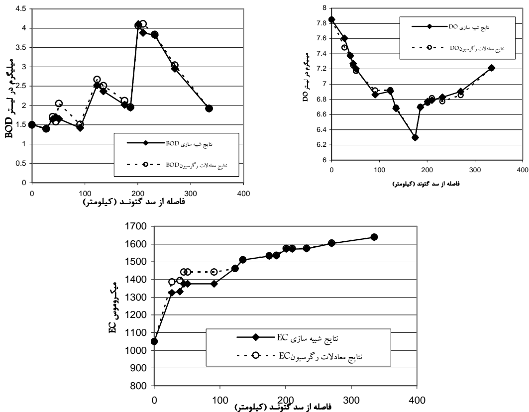
شکل ۸- نتایج شبیه سازی متغیرهای کیفی موردنظر در طول رودخانه با استفاده از مدل Qual2k و رابطه همبستگی خطی چندمتغیره
