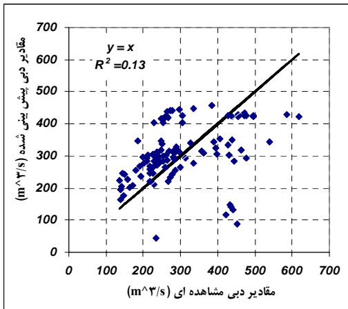
شکل ۳- مقادیر دبی مشاهده‌ای و دبی پیش‌بینی با روش اتورگرسو ساده
