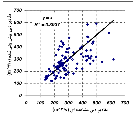
شکل ۲- مقادیر دبی مشاهده‌ای و دبی پیش‌بینی با روش پیشنهادی (تلفیق اتورگرسو و پیش‌بینی بارندگی)
