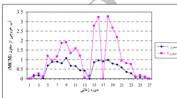
شکل ۱۴- نحوه آبیاری از مخازن R جهت آبیاری مزارع در مدل‌سازی الگوریتم ژنتیک برای سدهای پشت سر هم در شمال خراسان رضوی. حجم مخزن نیمه‌پر، رژیم بارندگی خشک و رژیم جریان رودخانه‌ای حداقل است.
