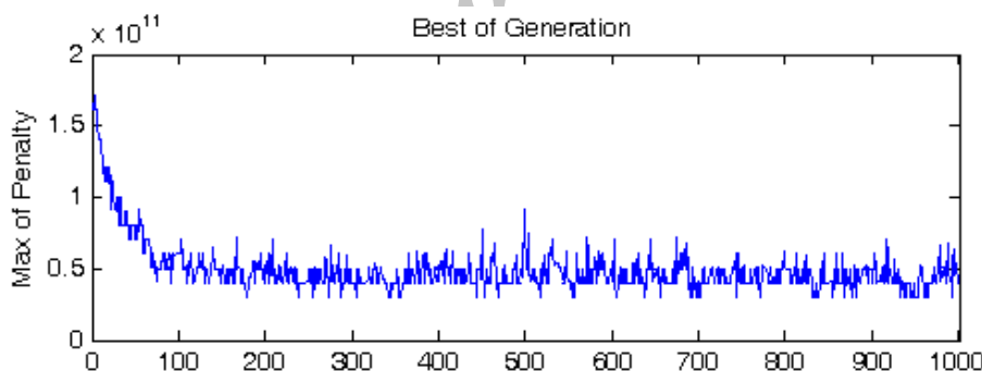
شکل ۵- حداکثر مجموع توابع جریمه در مدل‌سازی الگوریتم ژنتیک برای سدهای پشت سر هم در شمال خراسان رضوی (حجم مخزن نیمه پر، رژیم بارندگی خشک و رژیم جریان رودخانه‌ای حداقل است.)
